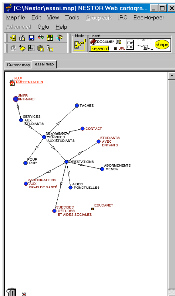
Figure 1 : la fenêtre «Map» dans Nestor qui permet de visualiser sous forme topographique l'itinéraire effectué pour visiter les pages d'un site WEB
